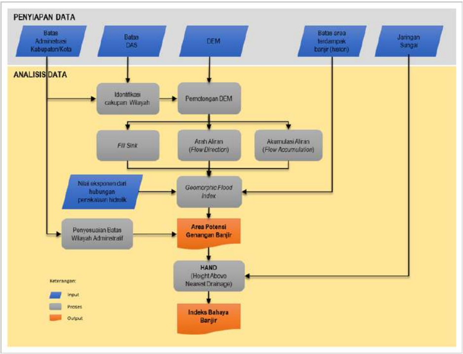
Gambar 3. 5 Alur Proses PembuatanIndeksBahayaBanjir
