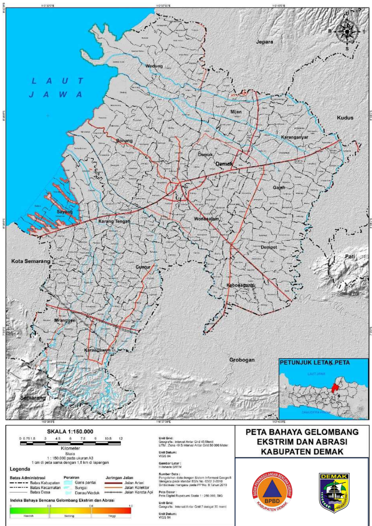
Gambar 3. 144 Peta Bahaya Bencana Gelombang Ekstrem dan Abrasi Kabupaten Demak
