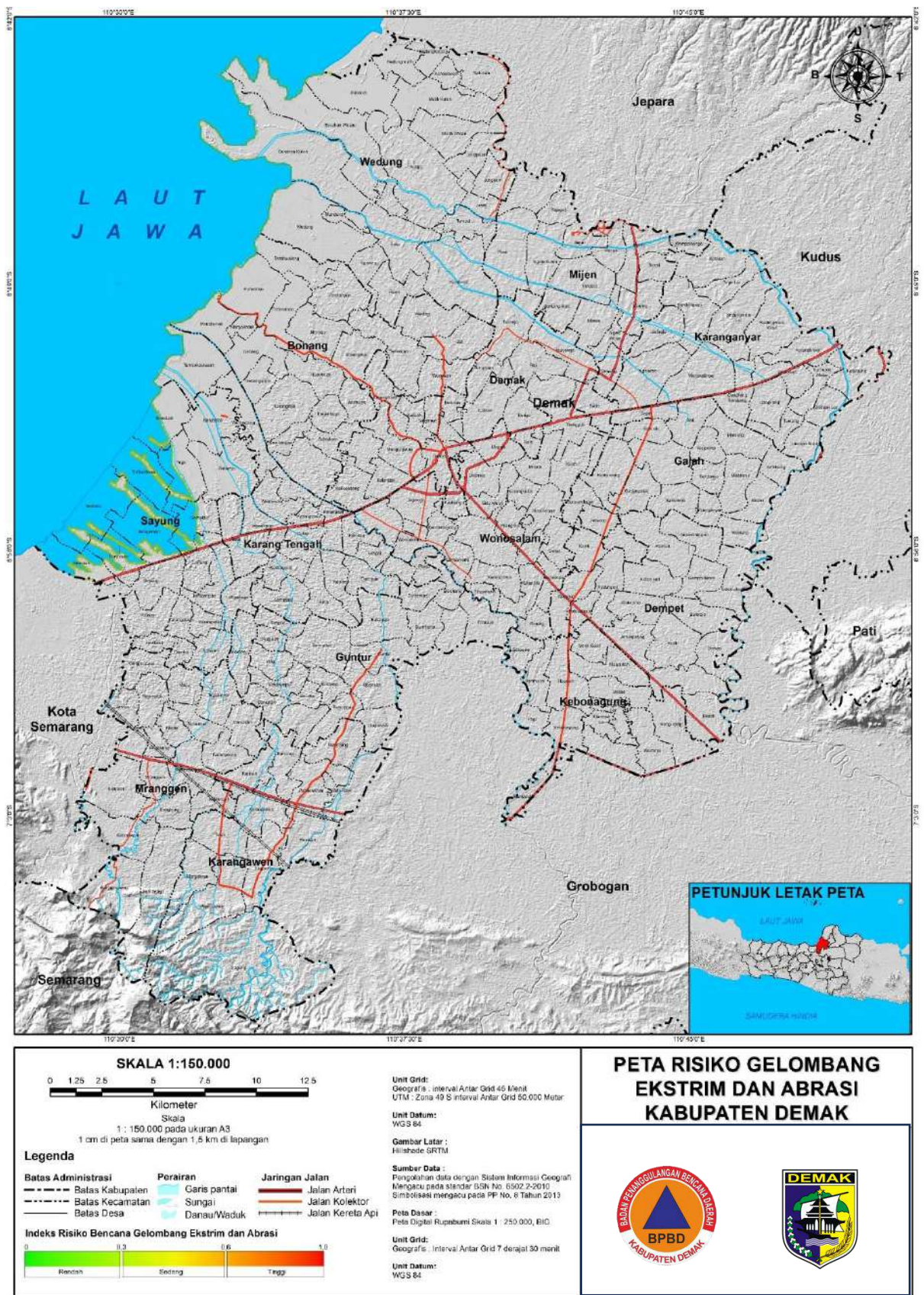
Gambar 3. 229 Peta Risiko Gelombang Ekstrem dan Abrasi Kabupaten Demak
