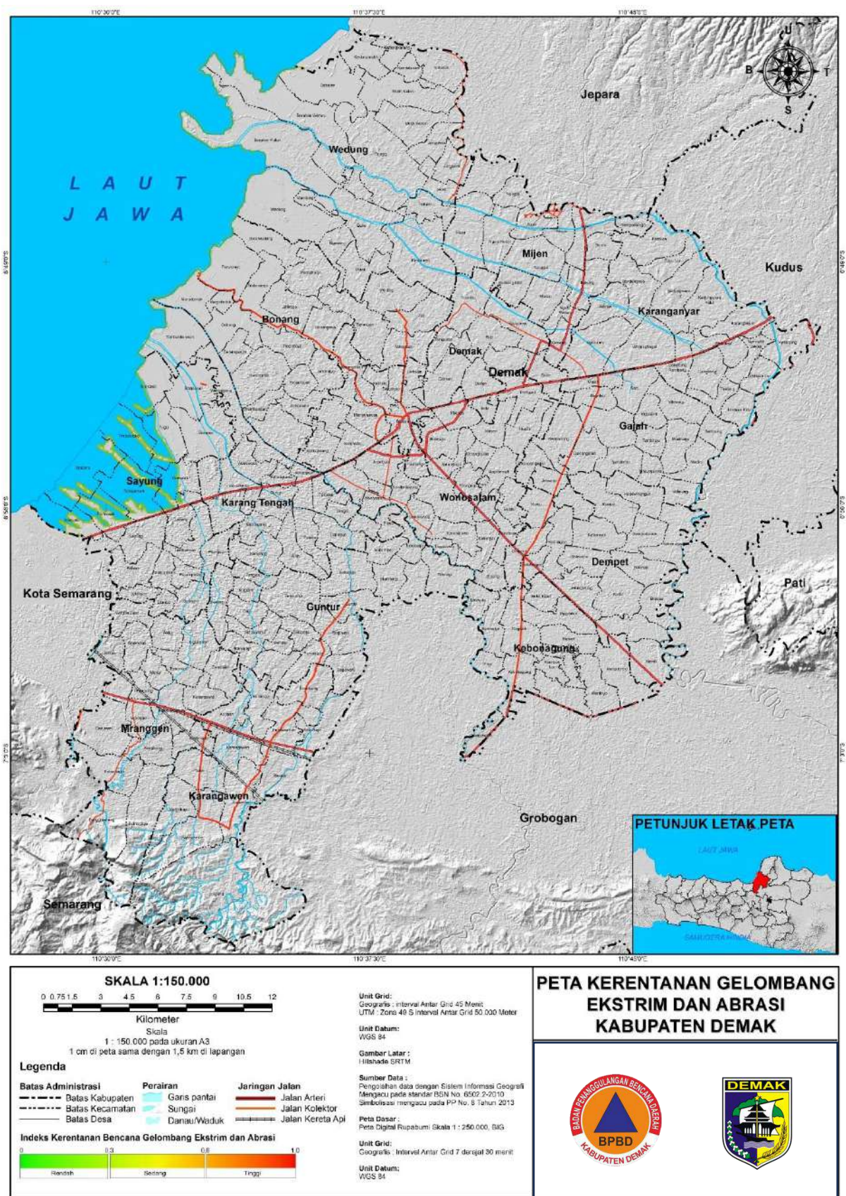
Gambar 3. 211 Peta Kerentanan Gelombang Ekstrem dan Abrasi Kabupaten Demak
