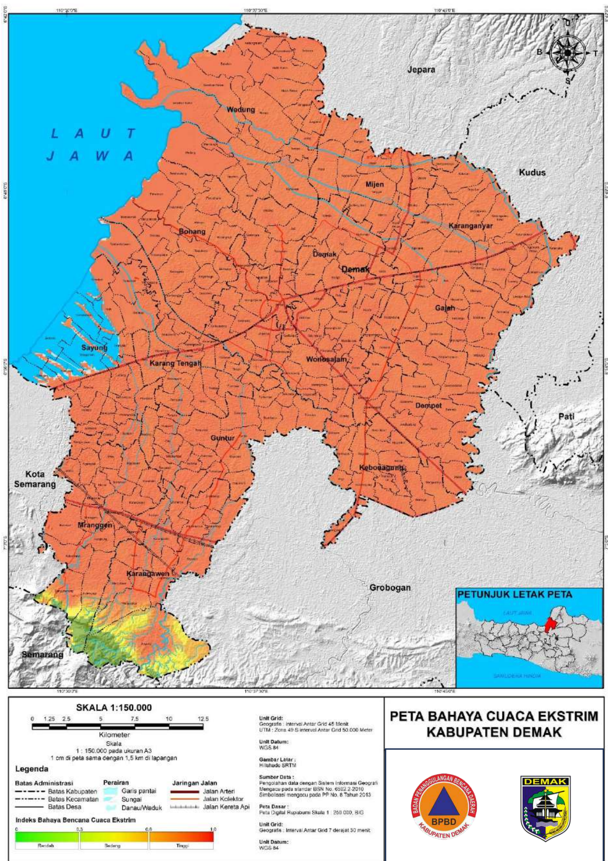
Gambar 3. 13 Peta Bahaya Bencana Cuaca Ekstrem Kabupaten Demak
