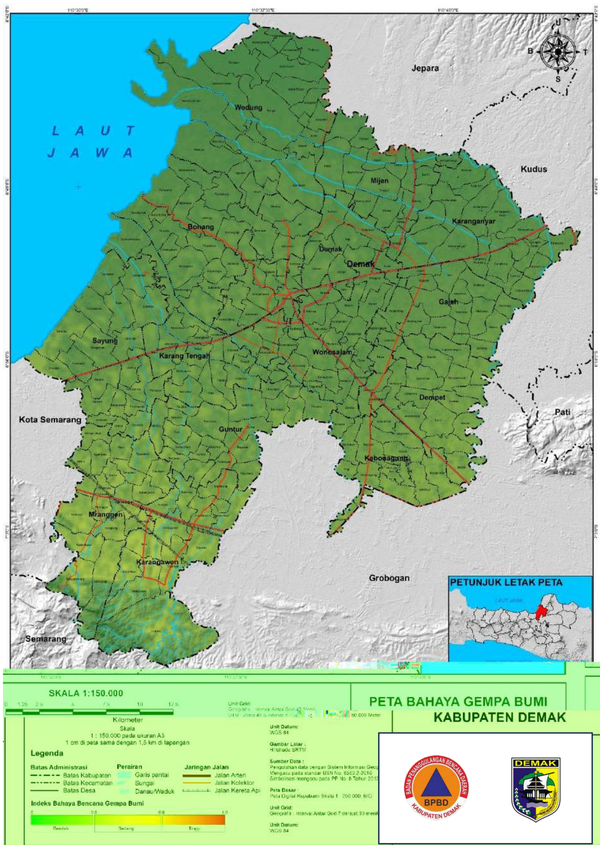
Gambar 3. 155 Peta Bahaya Bencana Gempa bumi Kabupaten Demak
