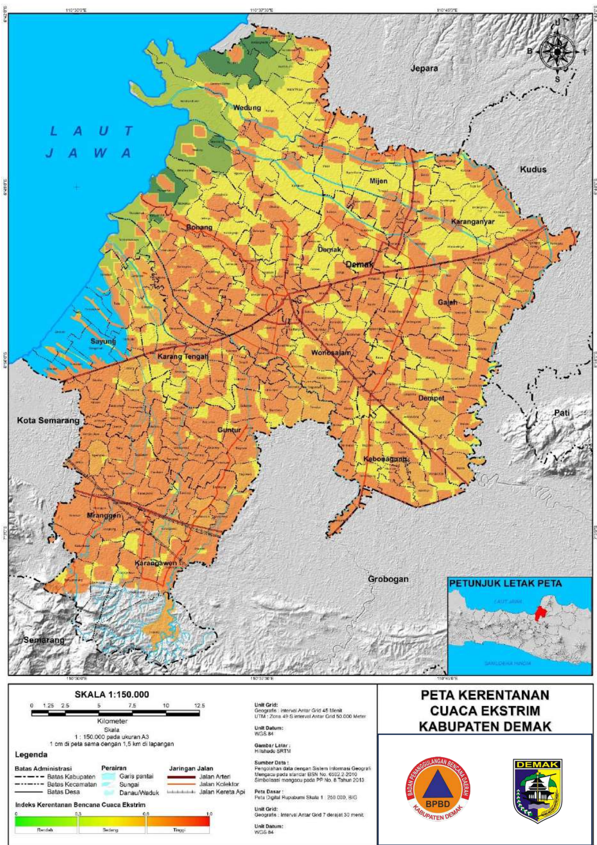
Gambar 3. 200 Peta Kerentanan Cuaca Ekstrem Kabupaten Demak
